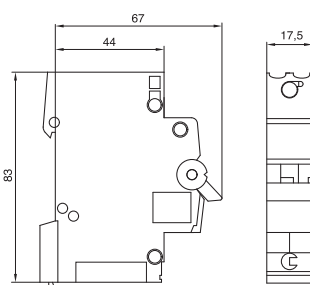
Чертеж с нанесенными размерами MB....A, MC...A
