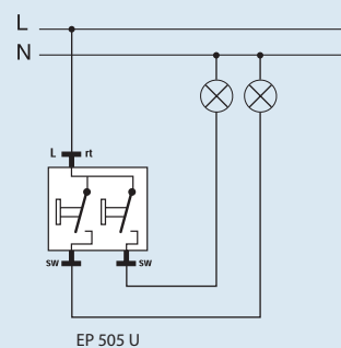
Двойной выключатель
