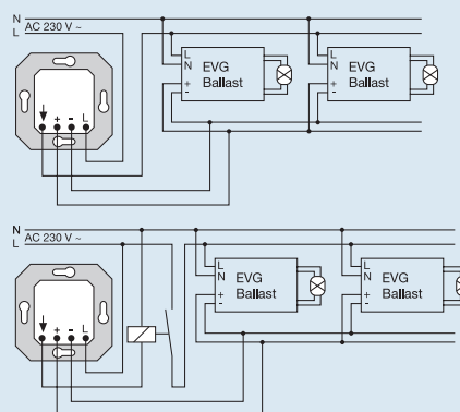
Управление люминесцентными лампами электронным потенциометром с выключателем (Арт. 240-10)
