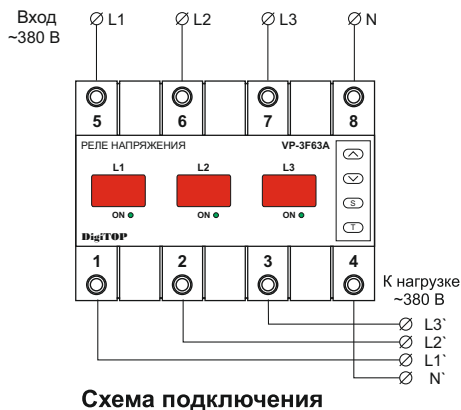
Схема подключения
