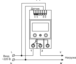
Схема подключения
