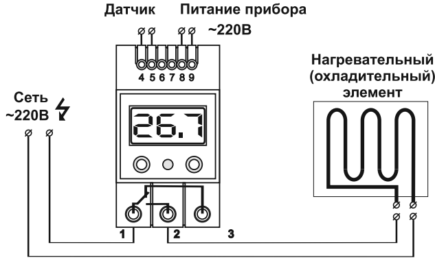
Назначение выводов
