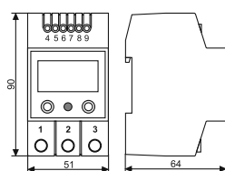
Габаритные размеры
