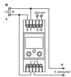
Схема подключения
