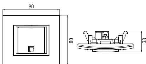
Технический чертеж выключателя
