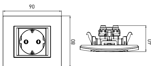
Технический чертеж розетки с заземлением
